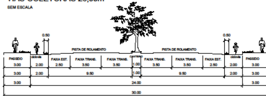
VIAS COLETORAS com CICLOVIAS - 30,00m
