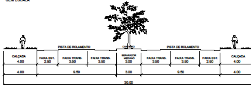
VIAS ARTERIAIS SECUNDÁRIAS - 30,00m
