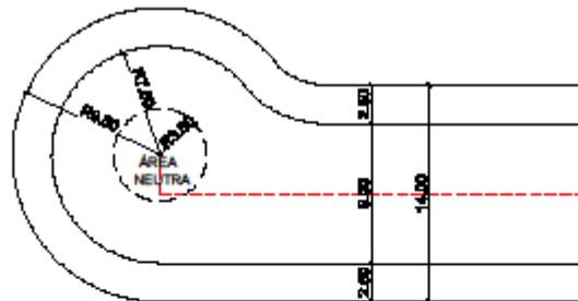
CUL DE SAC - VIAS LOCAIS - MODELO 2 LOTEAMENTOS/CONDÔMINIOS FECHADOS
