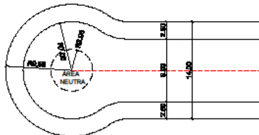
CUL DE SAC - VIAS LOCAIS - MODELO 1 LOTEAMENTOS/CONDÔMINIOS FECHADOS
