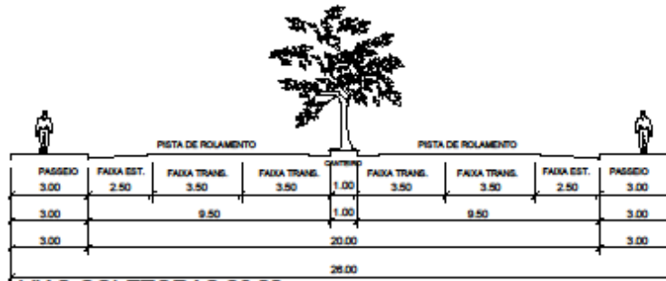
VIAS COLETORAS 26,00m
